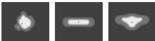
[P4] Spezielle Fussgängerüberweg Verteilung, rechte Verkehrsseite - 20x78° [T1] Typ I, Asymmetrisch, Seitenwurf - 111x48° [T2] Typ II, Asymmetrisch, Seitenwurf - 133x48°
