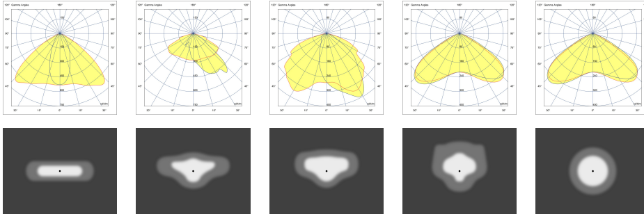
[T1] Tip I, Asimetrik, Kenara ışık atışı [T2] Tip II, Asimetrik, Kenara ışık atışı [T3] Tip III, Asimetrik, Kenara ışık atışı [T4] Tip IV, Asimetrik, İleri ışık atışı [T5] Tip V, Simetrik
